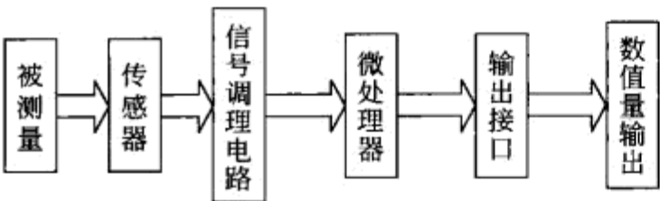
图 5-21 智能传感器典型结构
