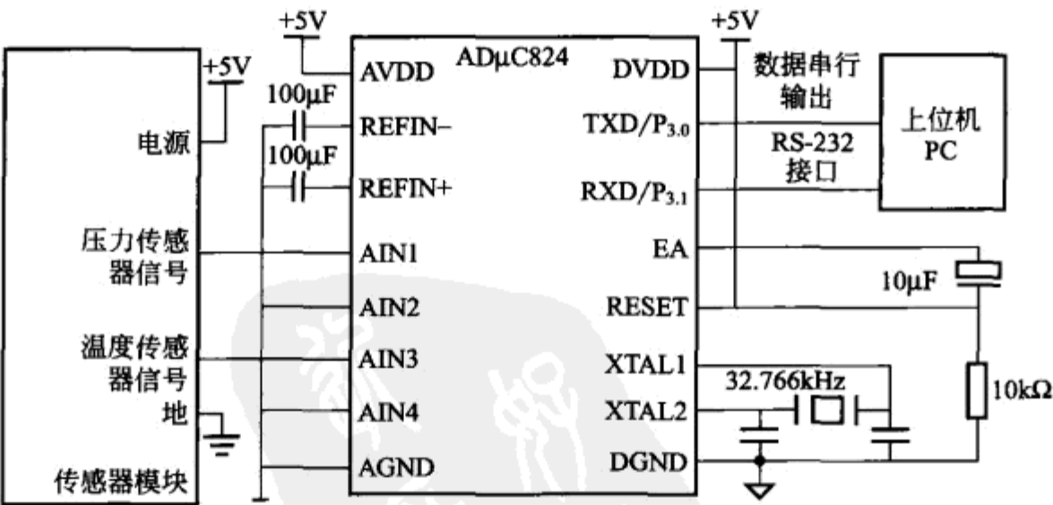
图 5-24 AD \mu C824 接口电路
